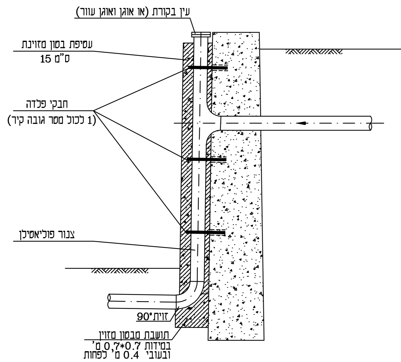
א. מפל גלוי מפלדה על קיר תומך
