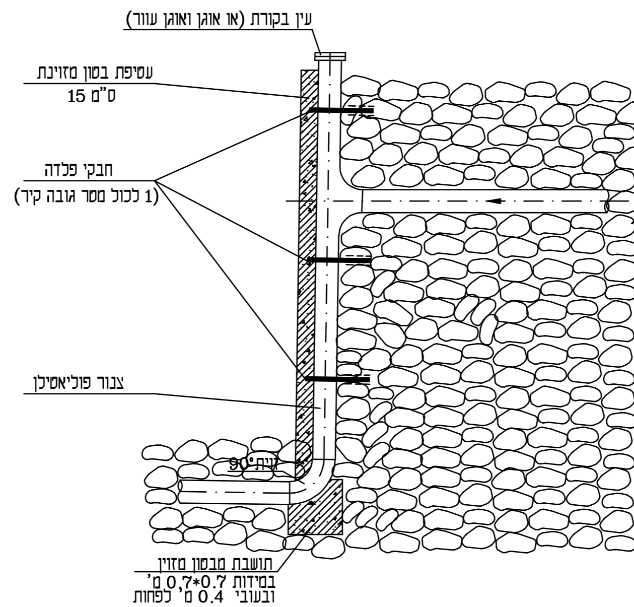
ב. מפל גלוי מפלדה על סלע חצוב
