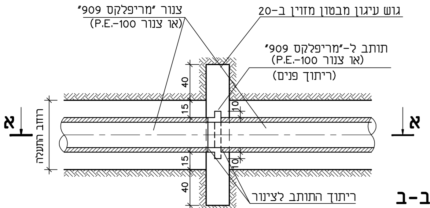
חציץ בטון על צינור פוליאטילן
