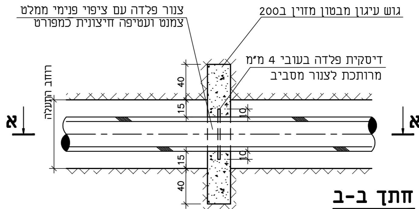
חציץ בטון על צינור פלדה
